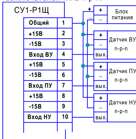
Рисунок Б5 - Схема подключения бесконтактных выключателей типа n-r-n при их питании от внешнего источника
