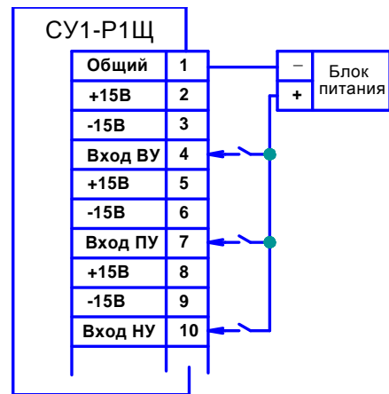
Рисунок Б8. Схема подключения «сухих» контактов с питанием от внешнего источника
