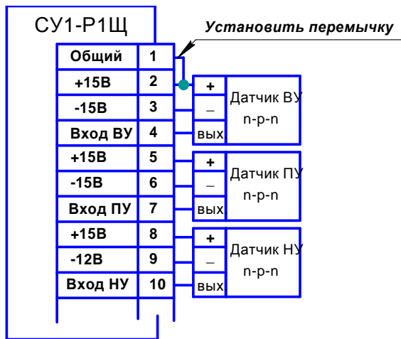
Рисунок Б3 - Схема подключения бесконтактных выключателей типа n-r-n.
