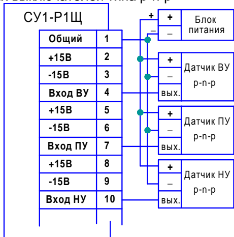
Рисунок Б4 - Схема подключения бесконтактных выключателей типа r-n-r при их питании от внешнего источника
