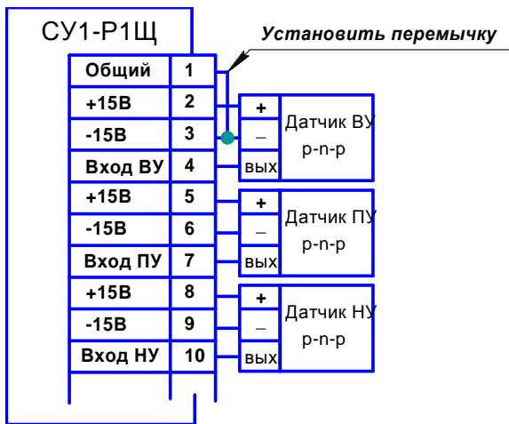
Рисунок Б2 - Схема подключения бесконтактных выключателей типа r-n-r
